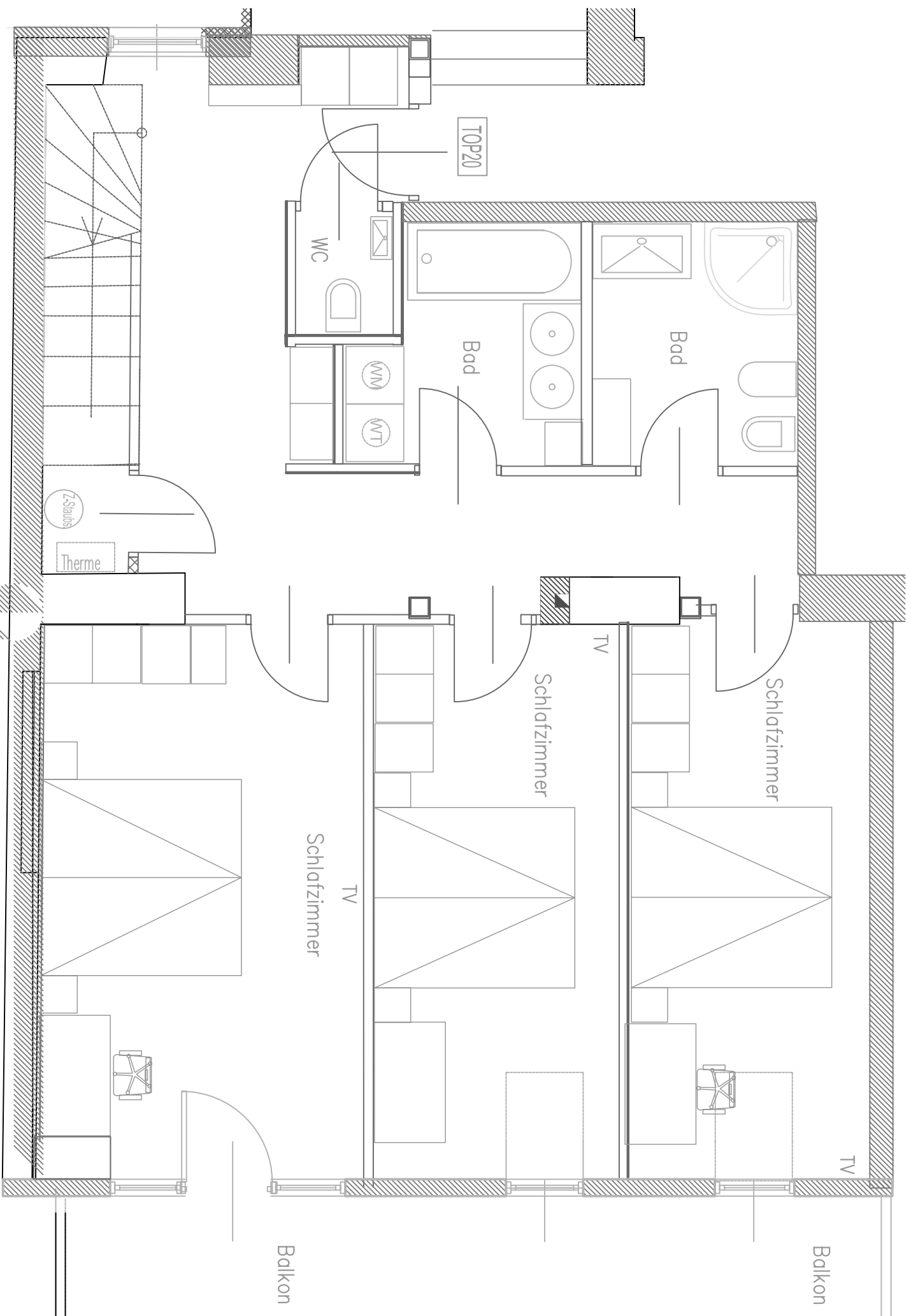
Thalistrasse 32, Stiege 2, Top 20, Untergeschoss
